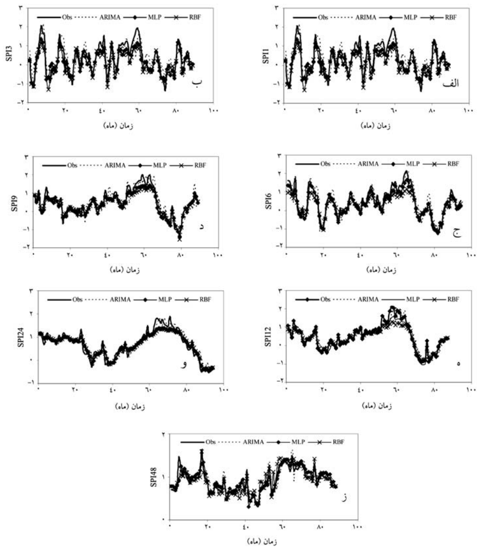
شکل ۶- مقایسه نتایج پیش‌بینی مدل‌های MLP, RBF, و ARIMA با مقادیر واقعی ایستگاه نوده،
