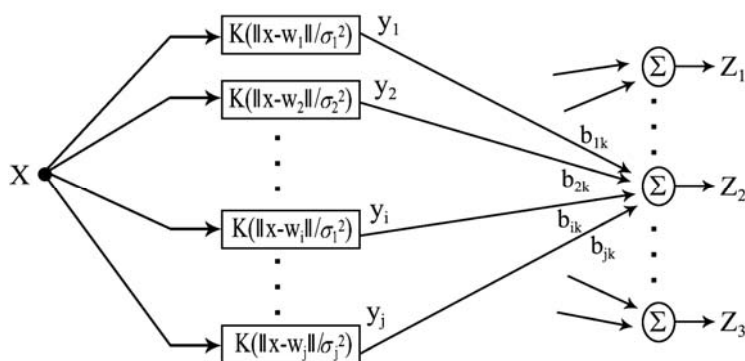
شکل ۲- شبکه عصبی مصنوعی تابع پایه‌ای شعاعی
