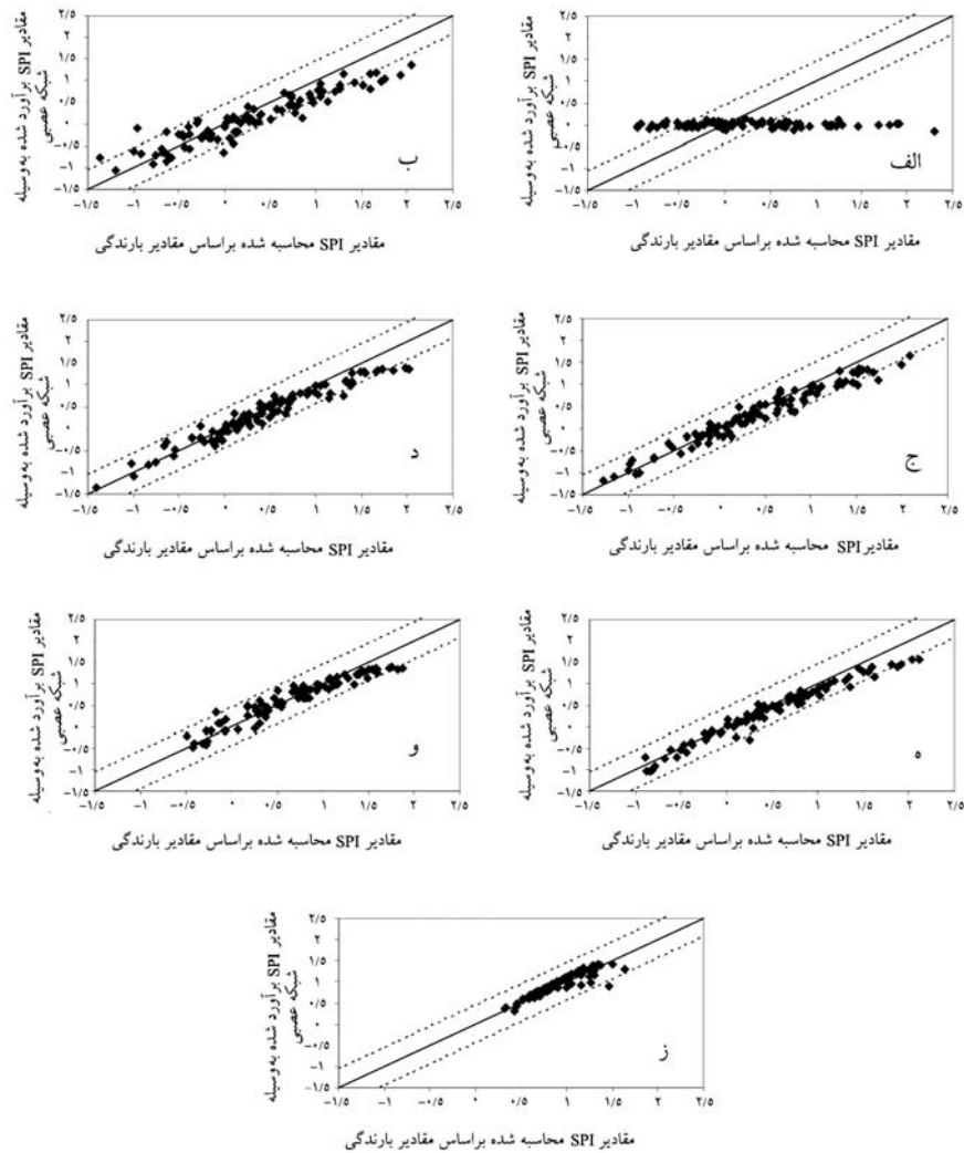
شکل ۳- مقایسه نتایج حاصل از به کارگیری شبکه عصبی مصنوعی MLP در دوره‌های مختلف زمانی SPI.
