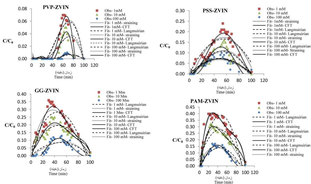
شکل ۴- منحنی رخنه اندازه‌گیری شده و برآورد شده نانوذرات آهن صفر ظرفیتی بر اساس قدرت یونی (غلظت نانوذرات ۲ گرم در لیتر، قدرت یونی ۱، ۱۰ و ۱۰۰ میلی‌مولار، داده‌های مشاهده‌ای = Obs، داده‌های برازش شده = Fit، تئوری پالایش = CFT، پالایش فیزیکی = straining، بلوکه شدن لانگمیر = Langmuirian).
