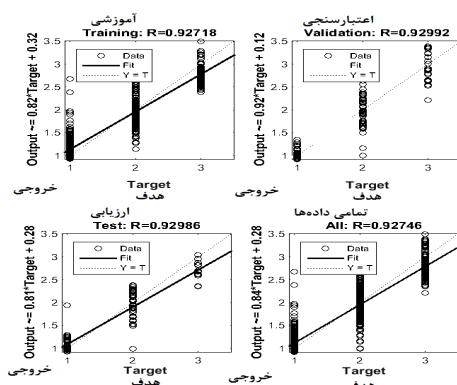
شکل ۵- نتایج رگرسیون خطی بین مقادیر تجربی و مدل شبکه عصبی مصنوعی.
