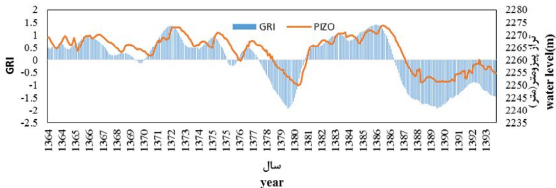
شکل ۵- تغییرات شاخص GRI در مقیاس زمانی ۱۲ ماهه در چاه مشاهده‌ای شماره شش در دوره زمانی ۹۴-۱۳۶۴. Figure 5. Variation of GRI index at 12-months time scale in piezometer No. 6 during 1985-2015.
