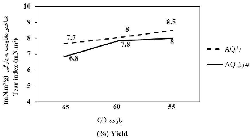
شکل ۶- اثر افزودن آنتراکینون بر شاخص مقاومت به پارگی کاغذ در بازده‌های مختلف.
