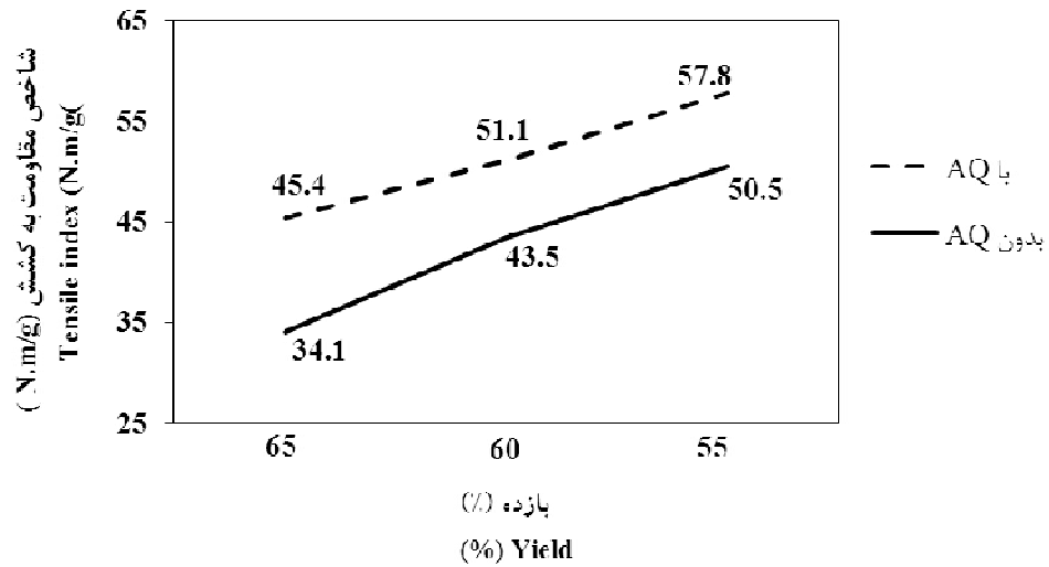
شکل ۵- اثر افزودن آنتراکینون بر شاخص مقاومت به کشش کاغذ در بازده‌های مختلف.
