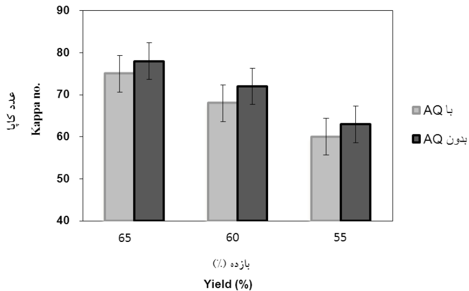
شکل ۱- اثر افزودن آنتراکینون بر عدد کاپای خمیر کاغذ NSSC در بازده‌های مختلف.
