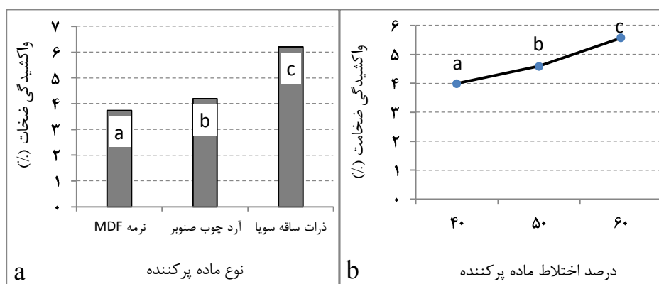
شکل ۳- اثر مستقل عوامل متغیر بر روی واكشیدگی ضخامت طولانی مدت.
