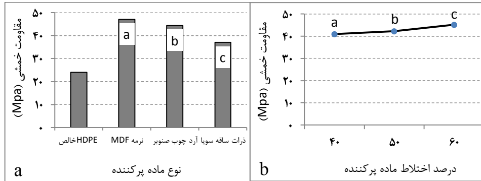
شکل ۴- اثر مستقل عوامل متغیر بر روی مقاومت خمشی.
