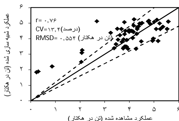
شکل ۳- مقادیر عملکرد مشاهده شده در برابر عملکرد شبیه‌سازی شده با مدل CropSyst در گندم. خطوط ممتد و نقطه چین به ترتیب نشان دهنده خطوط ۱:۱/۲، ۱:۱ و ۱:۰/۸ هستند.
