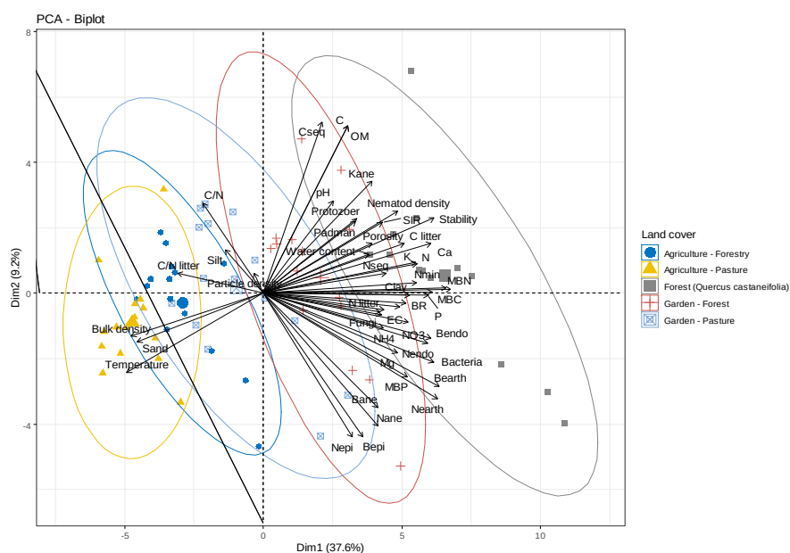
شکل ۱- ویژگی‌های لاشبرگ و خاک تحت کاربری‌های مورد مطالعه.
