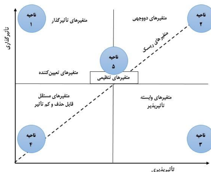
شکل ۲- صفحه پراکندگی تأثیرگذاری و تأثیرپذیری شاخص‌ها و موقعیت آن‌ها در روش تحلیل اثرات متقابل نرم‌افزار میک‌مک
