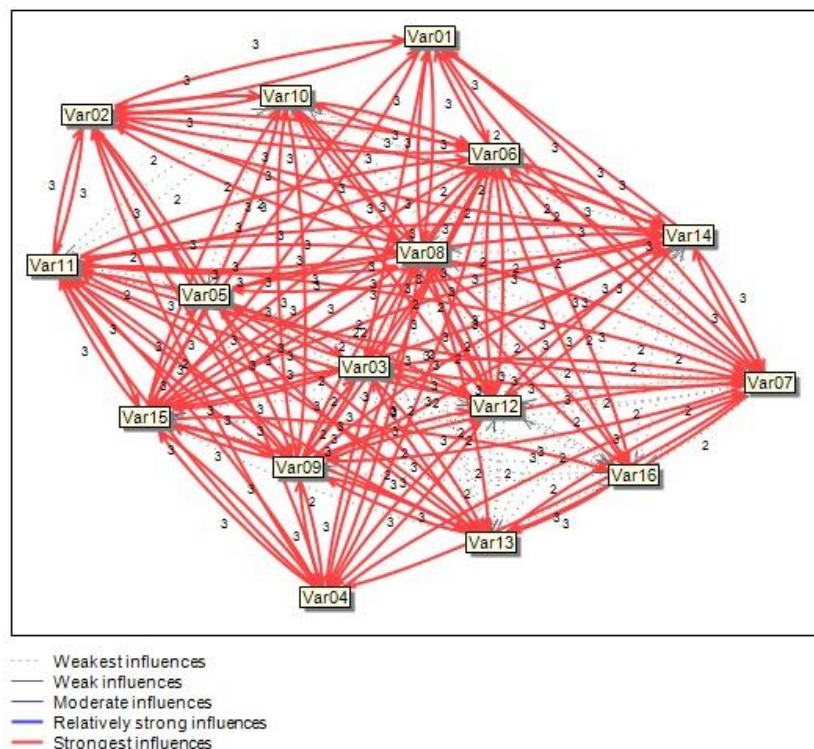
شکل ۴- تأثیرگذاری و تأثیرپذیری مستقیم شاخص‌ها بر یکدیگر
