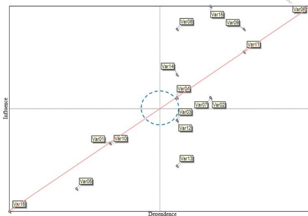
شکل ۳- اثرگذاری و اثرپذیری و پراکنش شاخص‌ها بر اساس اثرات مستقیم
